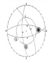
썰기 평사투영해석결과 - 63/173
